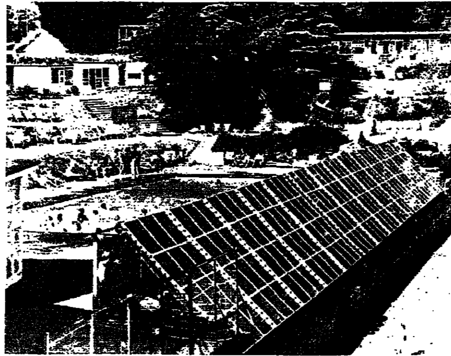
مجمع اجهزة امتصاص اشعة الشمس في احد فنادق الساحل الجنوبي من انكلترا . وهذا المجمع يستخدم لتسخين مياه حوض السباحة التابع لهذا الفندق بالإضافة الى تسخين المياه الجارية والمياه اللازمة لطبخ الفنادق وغرفة
